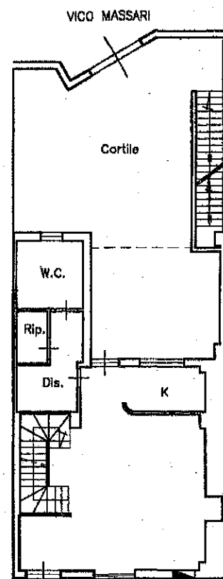
PIANTA PIANO TERRA H= 2.70
